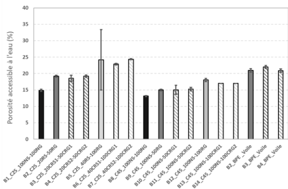
Figure 6. Porosité accessible à l'eau
