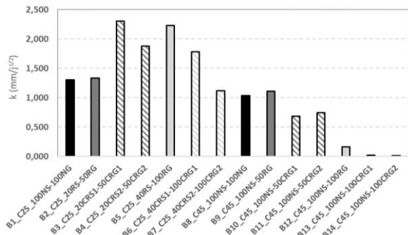
Figure 8. Vitesses de carbonatation accélérée
