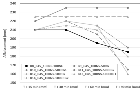
Figure 2. Affaissements mesurés pour les bétons C45/55
