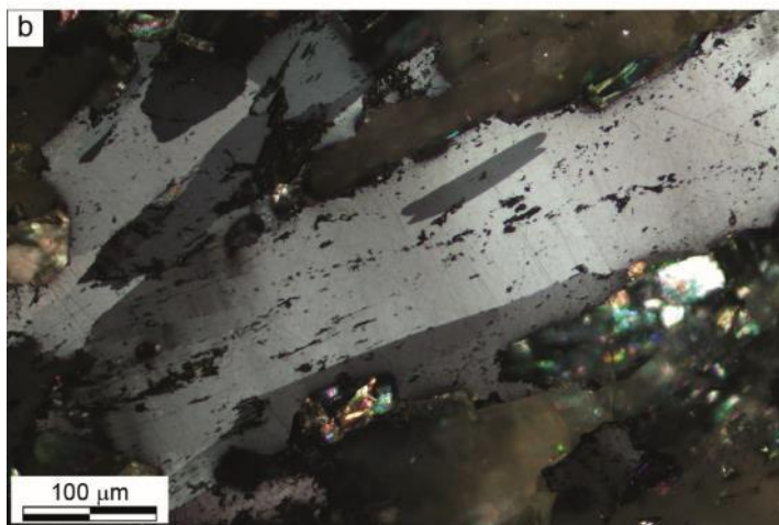
Figure 6. Microstructure de deux minerais du district de Brioude-Massiac vus en microscopie optique, lumière réfléchie, polariseurs croisés. a : la Croix-d'Astri, b : Luzer. © V. Thiéry, mars 2021.
