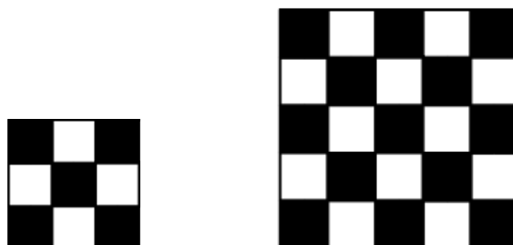
Figure 2. Les cases noires représentent le positionnement du lavabo pour lequel il est possible d'exhiber un pavage
