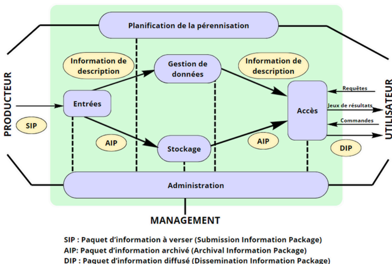
Figure 2 : Schéma d'ensemble du modèle fonctionnel OAIS
