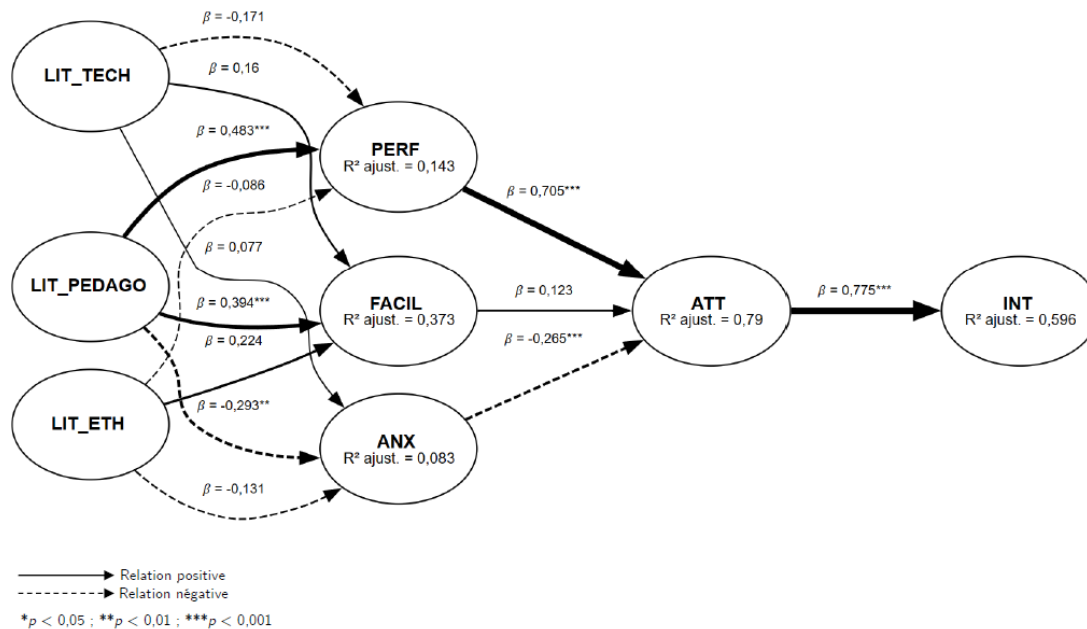
Figure 1. Estimation des paramètres du modèle d'équations structurelles
