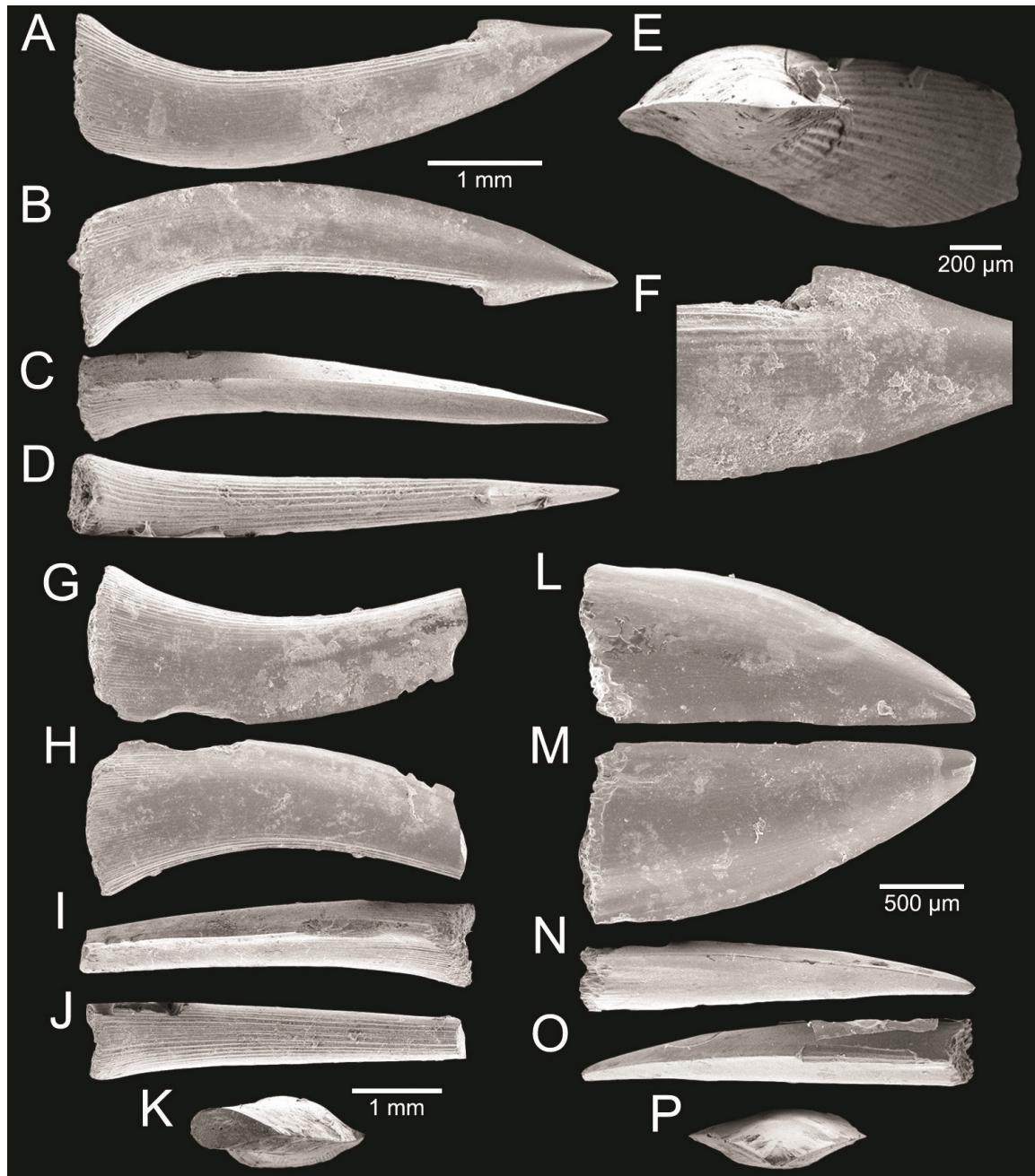
Figure 31. Trichiuridae indet. A–F specimen CUF-NKNY-2.1, anterior tooth in A, B lateral C anterior D posterior and E apical views F close-up of the tip of the tooth G–K specimen CUF-NKNY-2.2, anterior tooth in G, H lateral I anterior J posterior and K apical views L–P specimen CUF-NKNY-18.2, lateral tooth in L, M lateral N anterior O posterior and P apical views.
