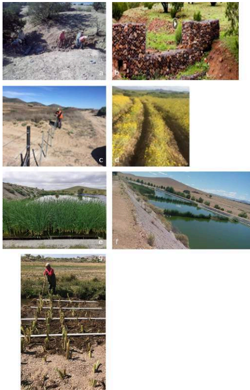
Figure 24 : a et b : Construction de barrages filtrants et de rétention des sédiments (Ejido Loma Pelona, 2019), c et d : Protection et restauration des sols, Ejido Centro Calles (50 ha) ; e et f : Zones humides hybrides dans la lagune d'oxydation aérobie de la station d'épuration d'Anahuac (zones humides fixes dans un substrat fixe de gravier-sable-terre) ; g : Zone humide en bandes fixes dans la zone de rejet des eaux usées à Anahuac
