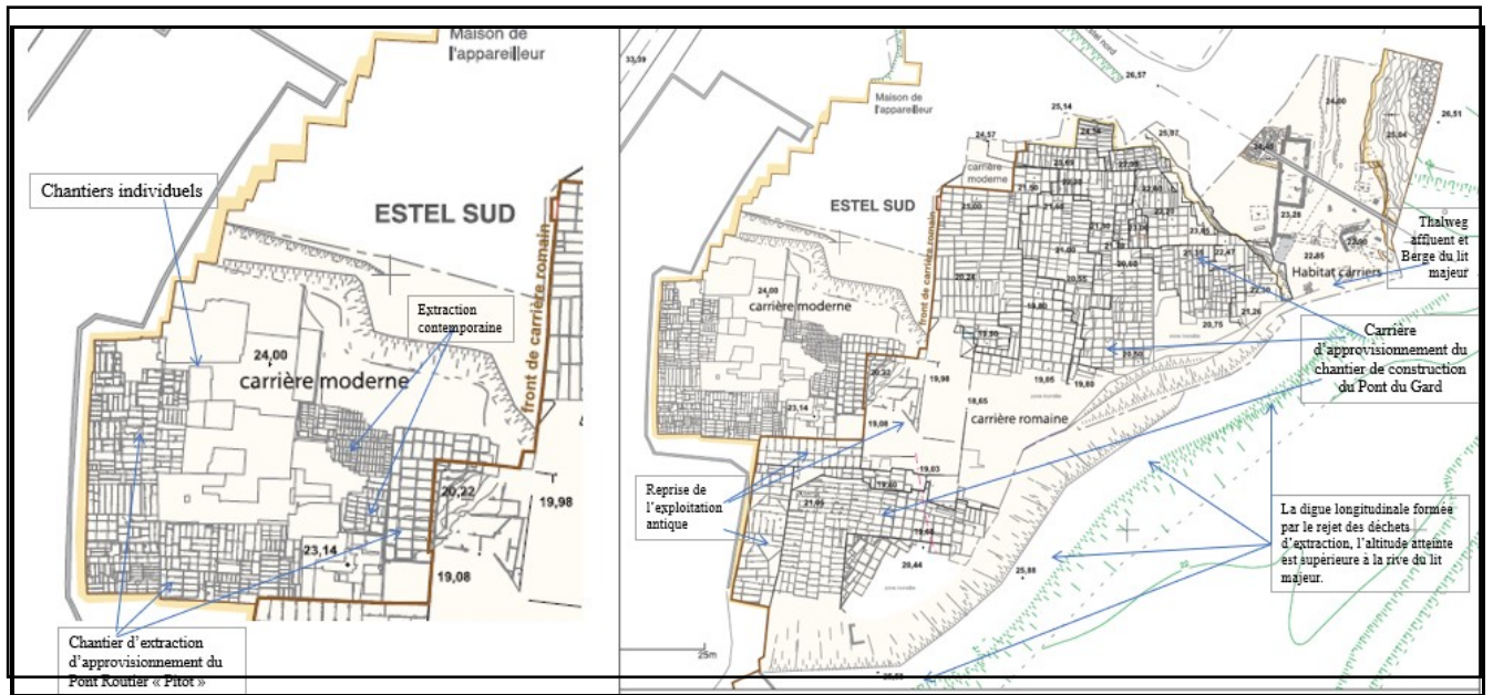
Fig. 17 – Répartition spatiale des séquences d'exploitations de la pierre de taille, du 1 er siècle à 1950. À noter, le front de taille d'abandon de l'exploitation antique. L'habitat des carriers, contemporain de la carrière antique initiale, est installé sur le comblement protohistorique du thalweg de Font Grasse au nord du site. (Topographie, infographie, V. Vachon, Inrap, 2002 ; Vacca-Goutoulli 2006).
