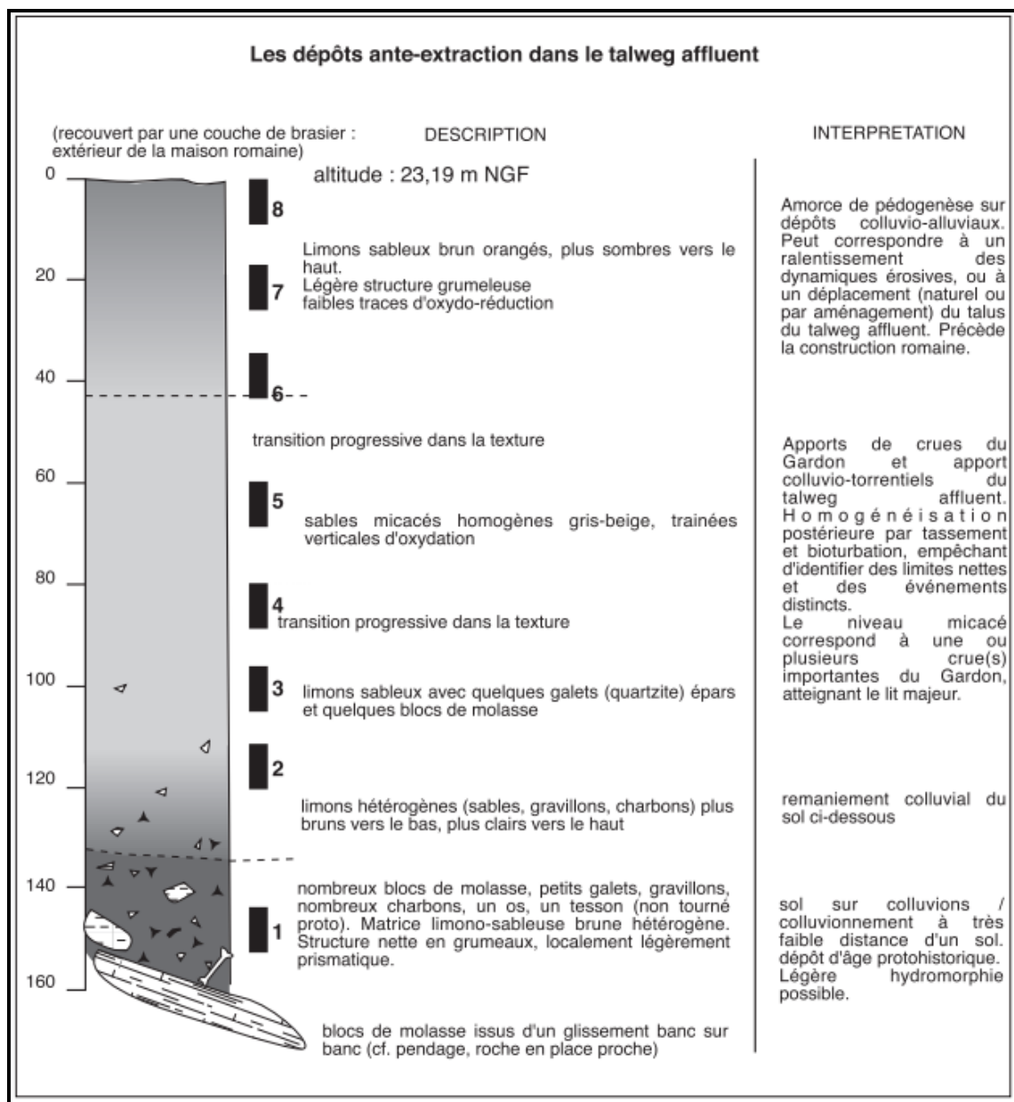
Fig. 6 – Hydromorphologie antérieure à l'extraction antique initiale. Coupe effectuée sous les fondations de la dernière maison de carrier à l'est de l'habitat en lanière, milieu du I er siècle (Bruneton 2002 ; Vacca-Goutoulli, Bruneton 2004).
