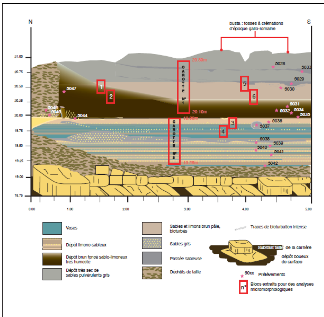
Fig. 13 – Coupe du remplissage du chemin d'accès à la reprise de l'exploitation dans la seconde moitié du I er siècle. (Pascale Chevillot, Inrap 2001, infographie : Ribes, 2001 ; Vacca-Goutoulli 2002).
