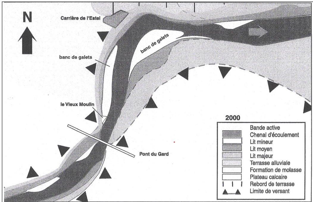
Fig. 5 – La bande active du Gardon au niveau du Pont du Gard et du site de l'Estel. Étude géomorphologique du lit mineur de la rivière. Emanuel Ribes, document extrait du mémoire de DEA, sous la direction de Mireille Provansal, CEREGE (université Aix-Marseille, 2001).
