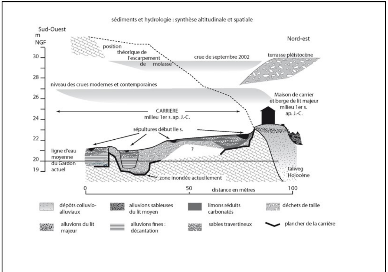
Fig. 4 – Coupe synthétique altitudinale et spatiale du site de l'Estel sud, 1 er siècle (Bruneton 2002 ; Vacca-Goutoulli, Bruneton 2004).
