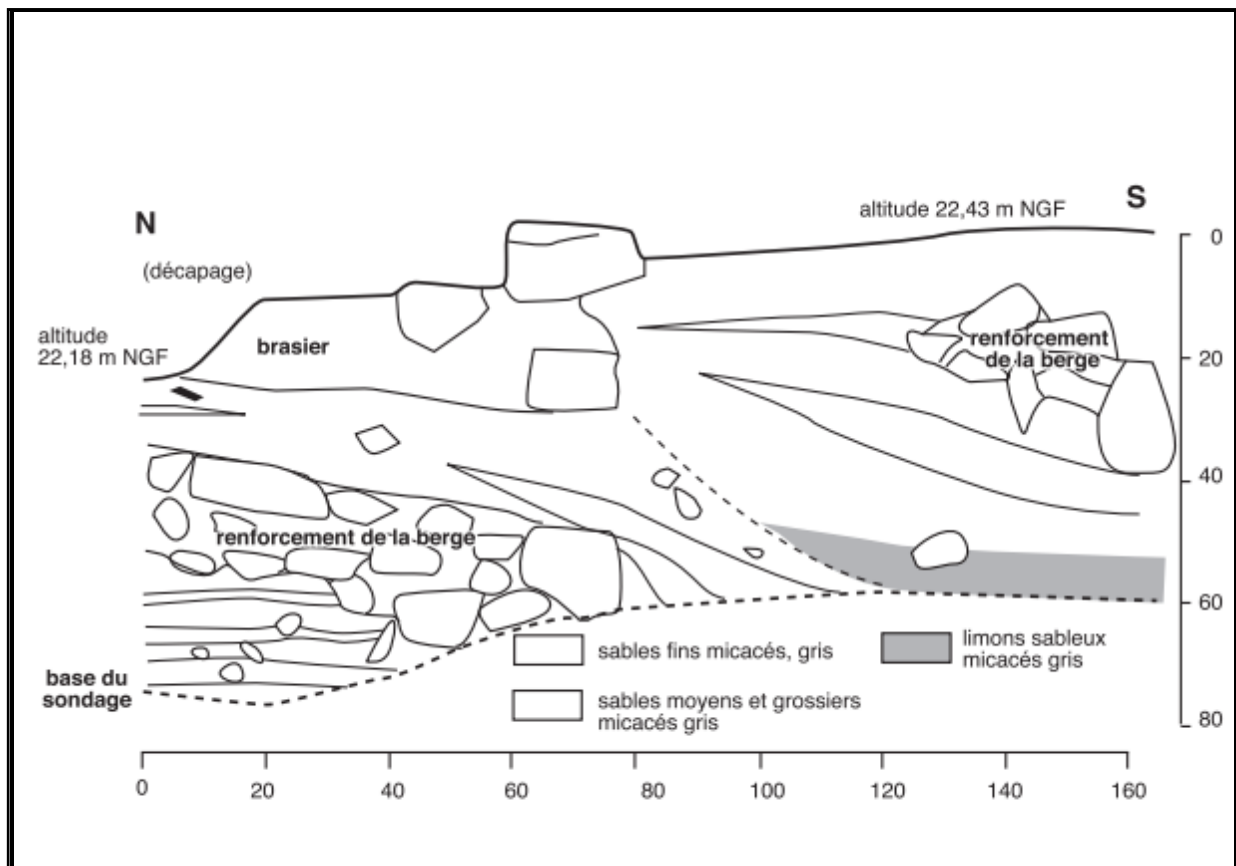
Fig. 9 – À l'aval et en contre-bas de l'habitat de carriers, coupe de la berge du lit majeur du Gardon, au confluent avec Font Grasse. Renforcements successifs de la berge avec des déchets de l'extraction initiale, le talus de la berge est progressivement repoussé vers le sud/sud-est. (Coupe : Bruneton, 2002 ; Vacca-Goutoulli, Bruneton 2004).
