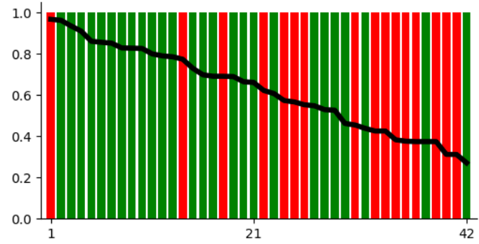
GPT-4
