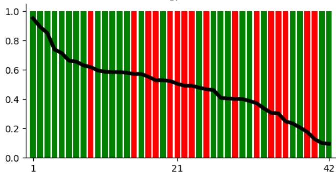
gpt4
