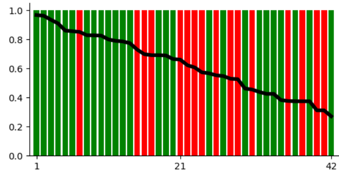
Llama-2
