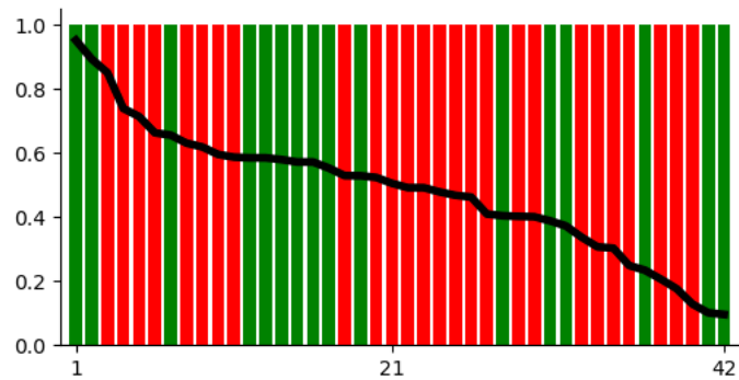
llama2
