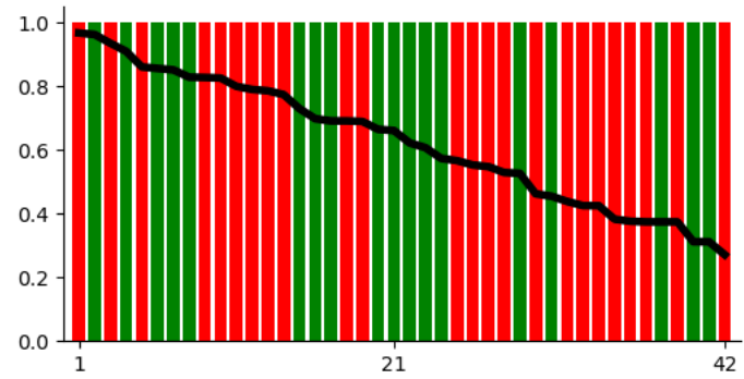
GPT-3.5
