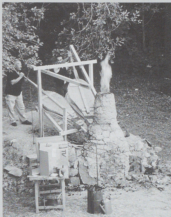
Reconstitution de bas-fourneau soit gallo-romain, soit du haut Moyen Âge, qui permet, en réduction directe (minerai oxydé-métal), d'obtenir un bloc (massiau) qu'il faudra ensuite épurer par martelage à la forge.
