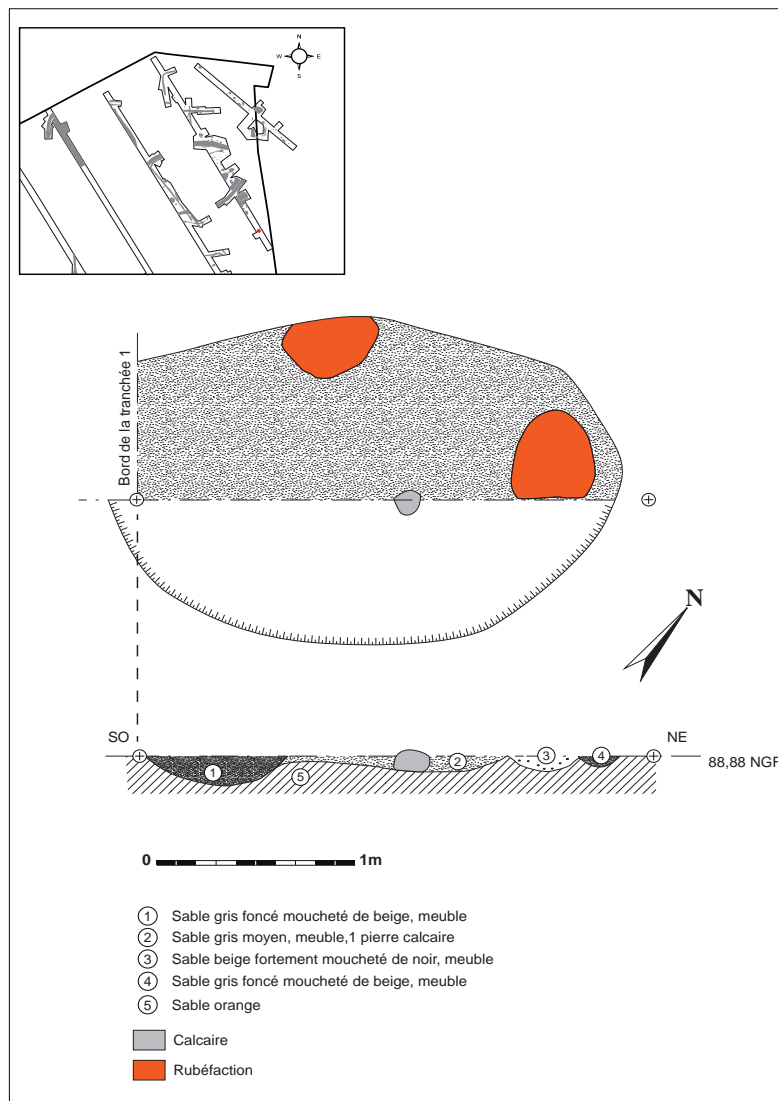
Fig. 60 : Plan et coupe de la fosse 033
