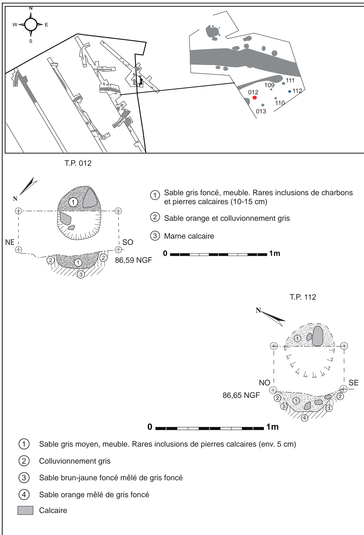
Fig. 27 : Relevé en plan et en coupe des trous de poteau 012 et 112
