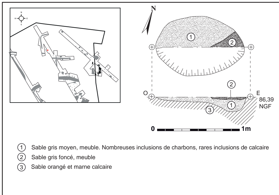
Fig. 29 : Relevé en plan et en coupe de la fosse 003
