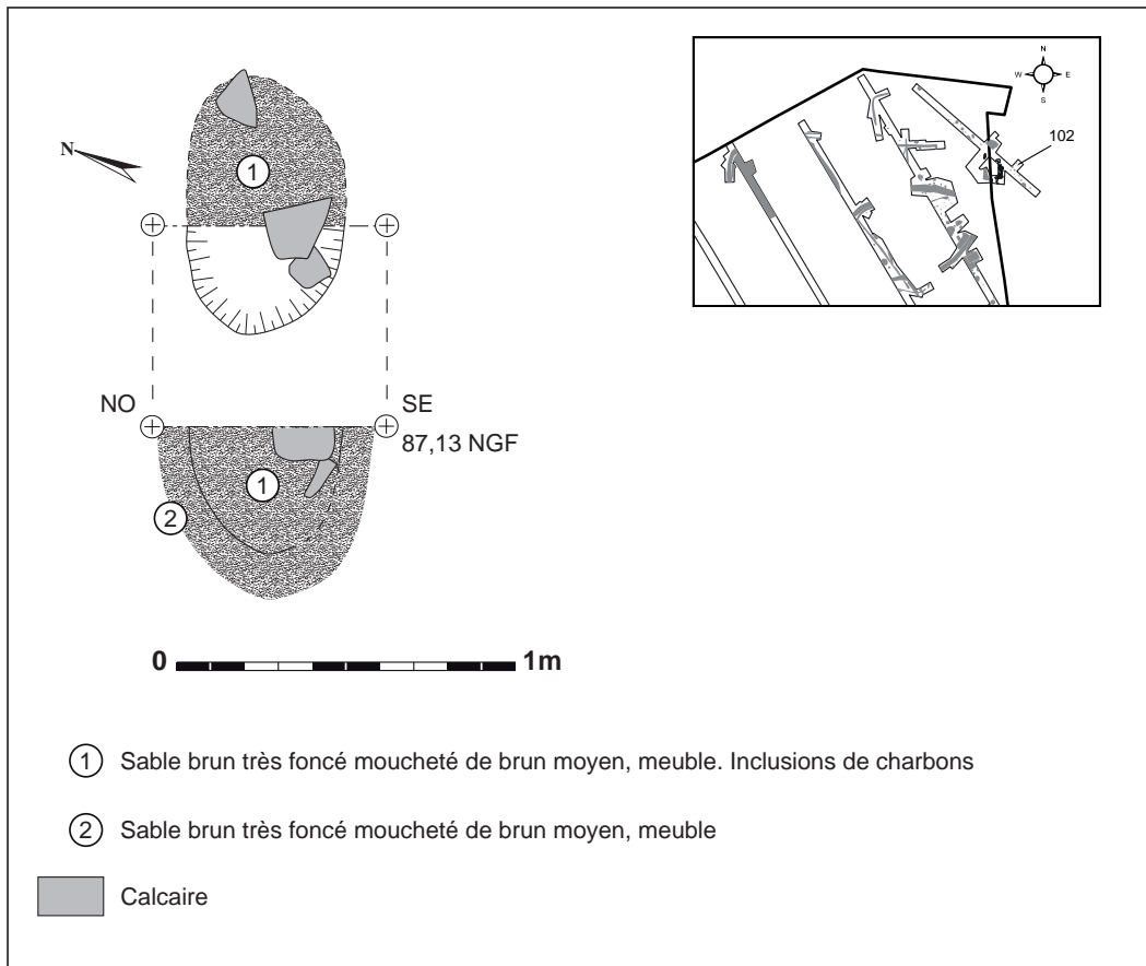
Fig. 67 : Le trou de poteau 102
