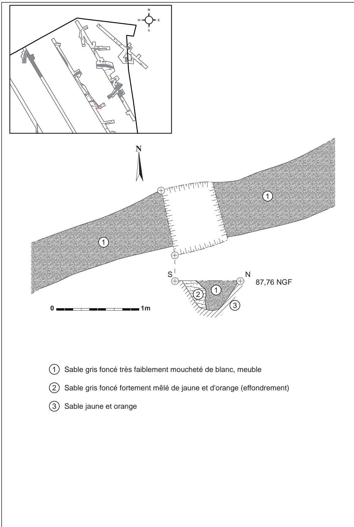
Fig. 42 : Plan et coupe du fossé 055
