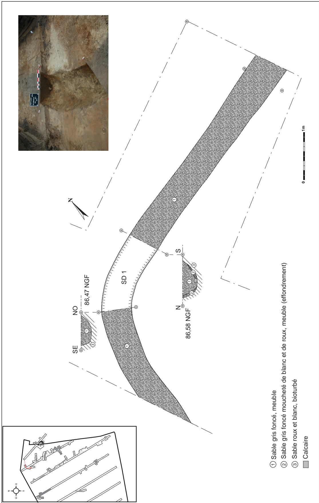
Fig. 16 : Le fossé 001, relevé en plan et coupe, photo de la coupe N/S
