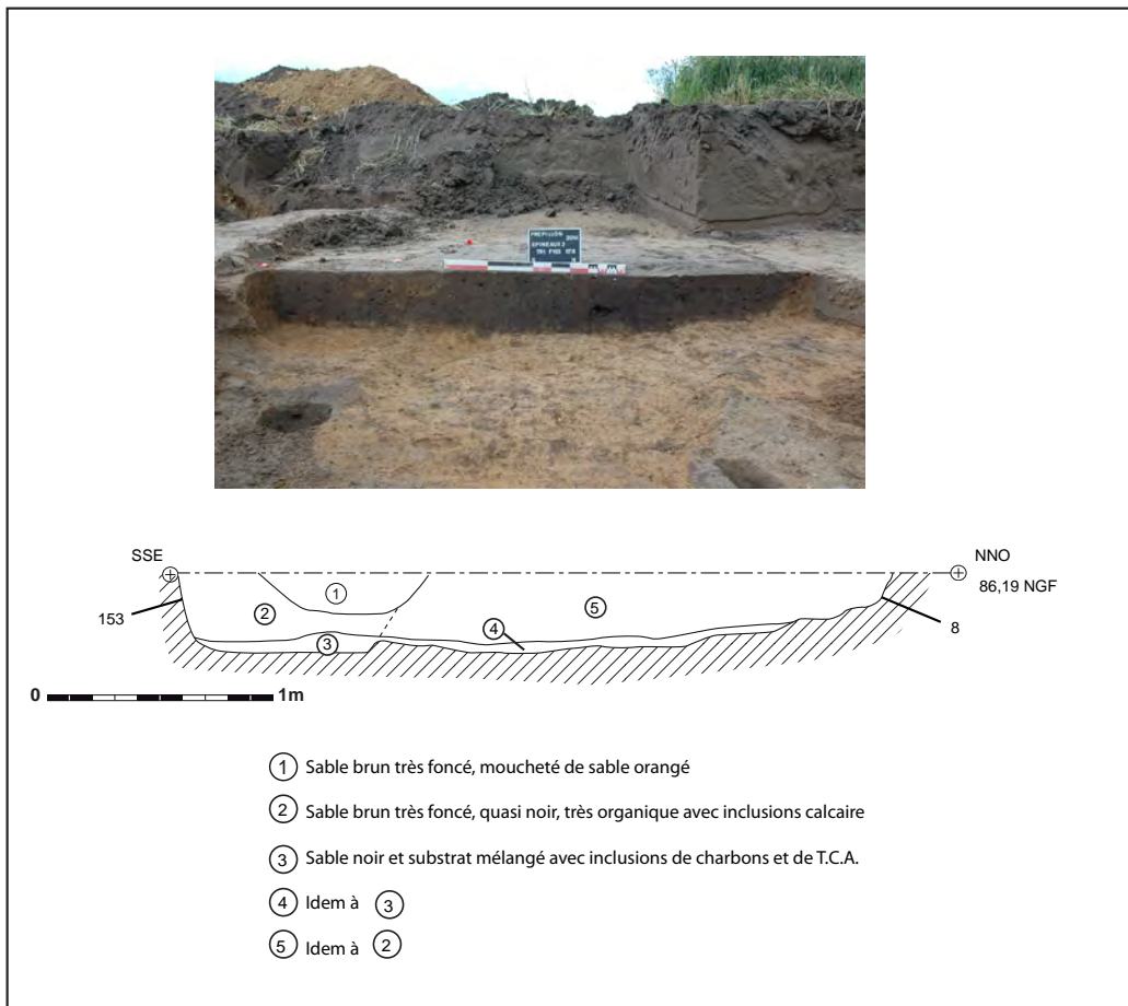
Fig. 35 : Coupe du fond de cabane 008 et de la fosse 153
