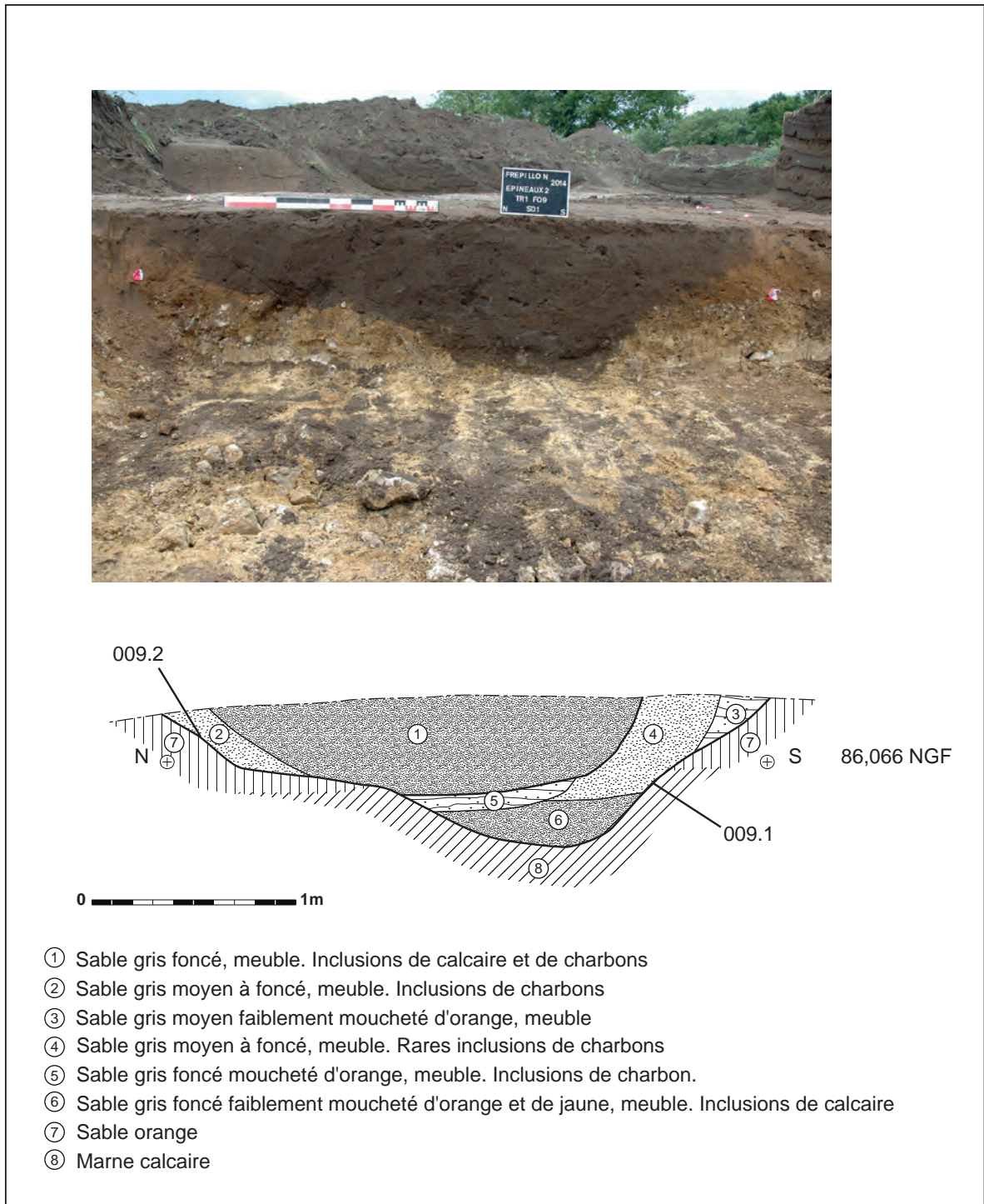
Fig. 40 : Cliché et coupe du tronçon de fossé 009
