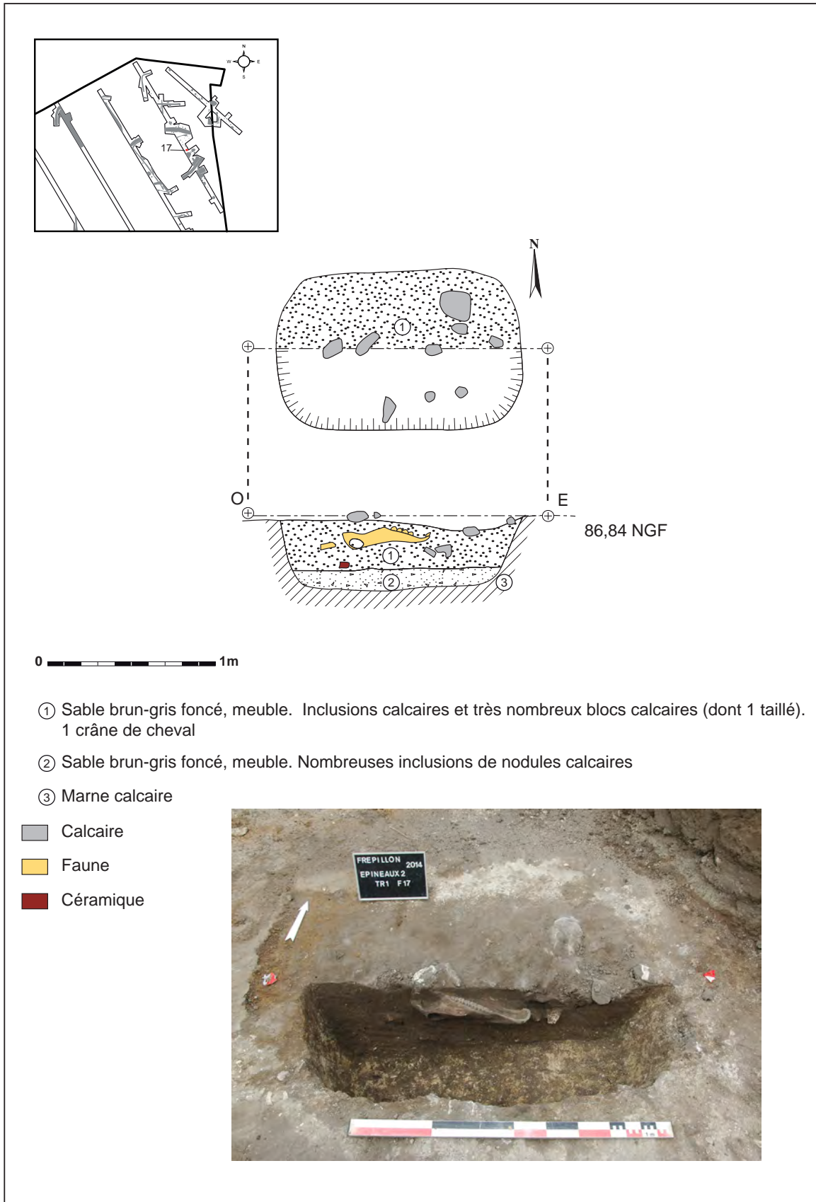
Fig. 59 : Plan, coupe et cliché de la fosse 017
