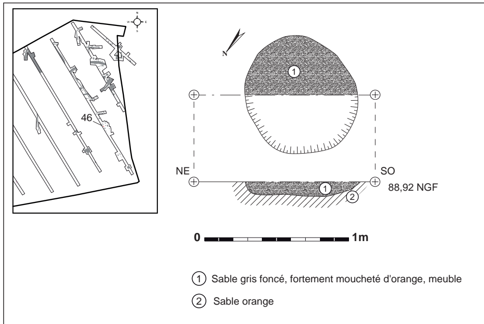
Fig. 63 : Plan et coupe de la fosse 046
