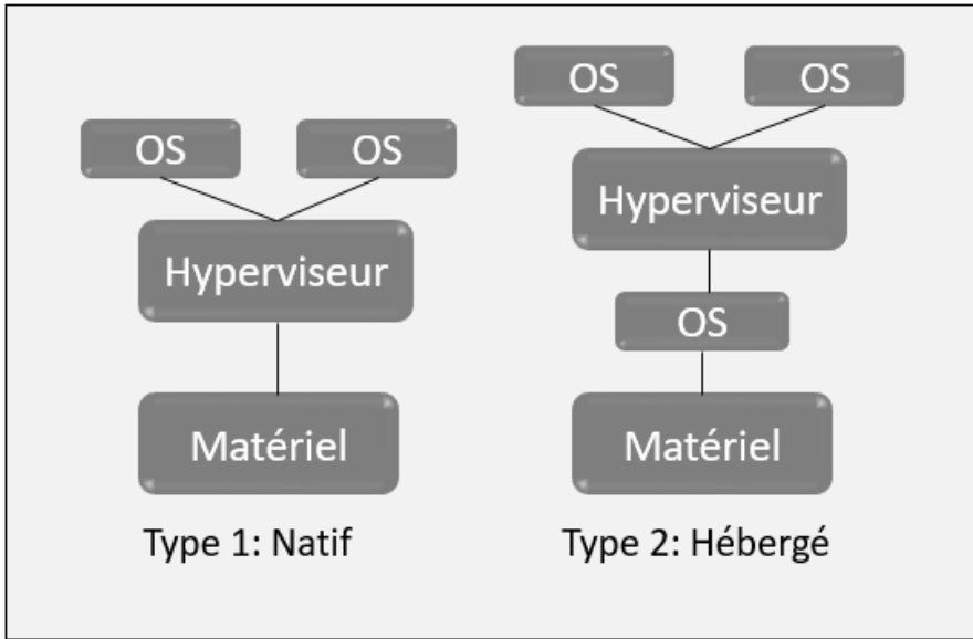
Figure 5. Hyperviseur type 1 et hyperviseur type 2
