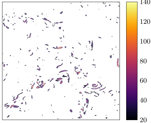
(b) |\omega| > \langle |\omega| \rangle + 2\sigma
