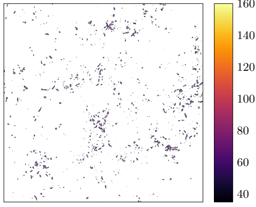
(d) |\omega| > \langle |\omega| \rangle + 2\sigma
