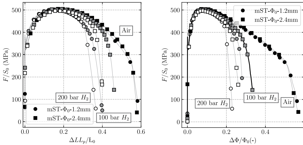
(a): F/S_0 - \Delta LL_p/L_0 plot.
