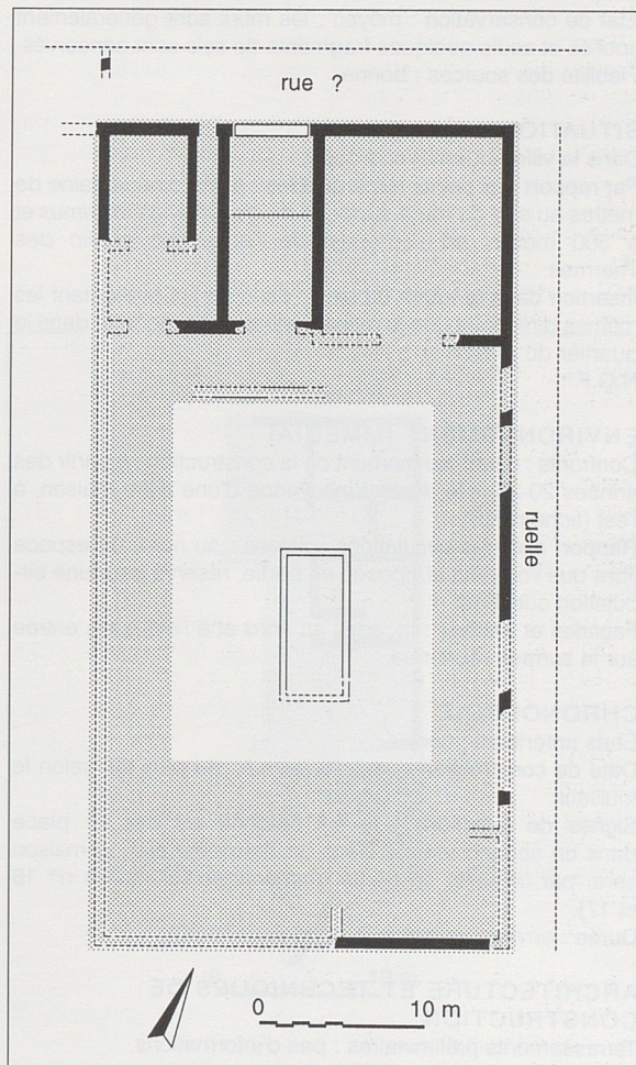
plan restitué
