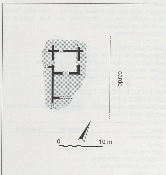
plan restitué
