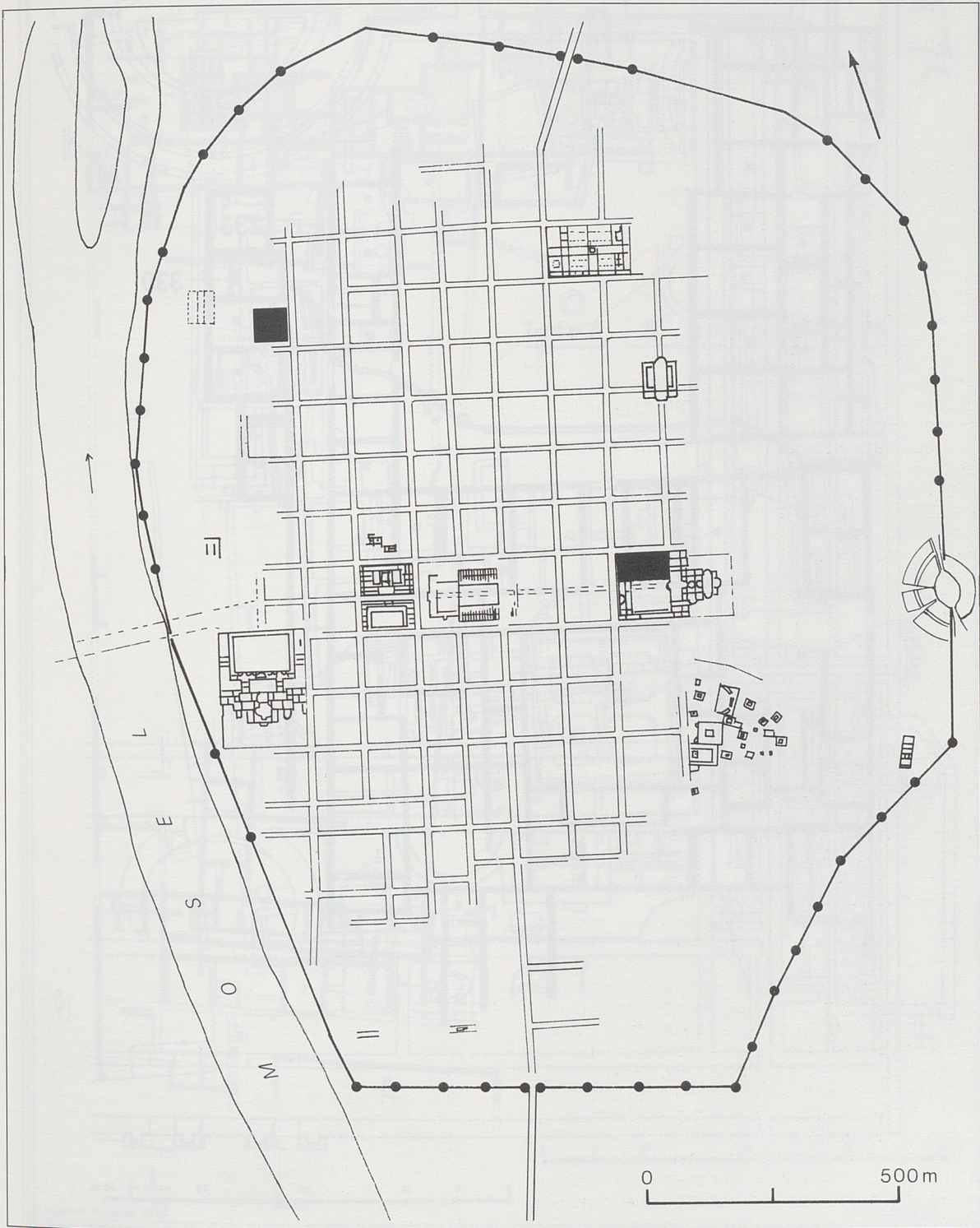
2. Plan de Trèves avec localisation des quartiers d'habitat sous les thermes impériaux et à Saint-Irmine.
