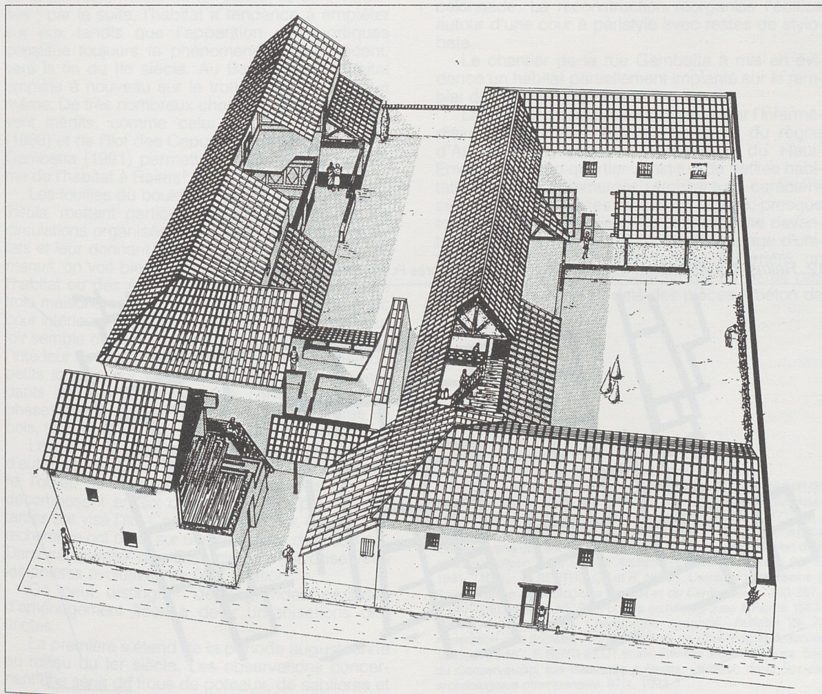
11. Amiens, Palais des Sports: reconstitution de deux maisons de dimensions moyennes (d'après E. Binet).
