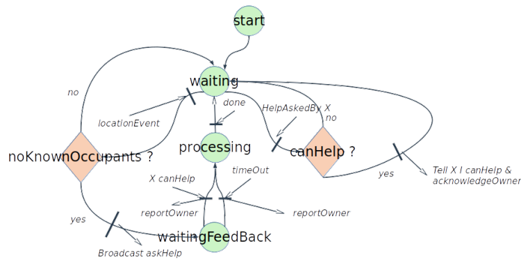
FIGURE 3 – Comportement d’un agent de maison.
