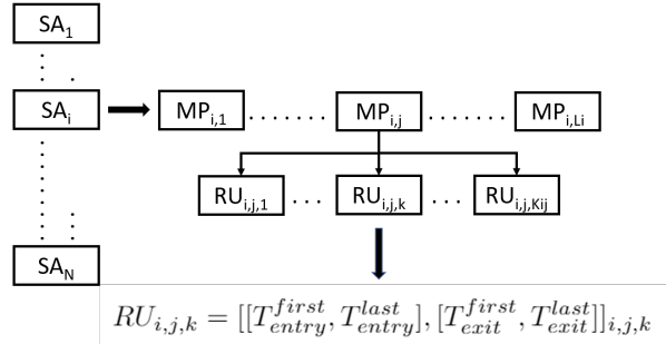
FIGURE 2 – Sortie de L-ADRIP
