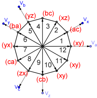
Fig. 8. Plan complexe avec 12 vecteurs de l'étage redresseur
