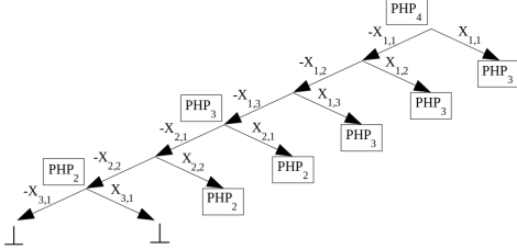
FIGURE 2 – Branche unique attendue en résolvant le problème PHP_4 . Les propagations ont été omises.
