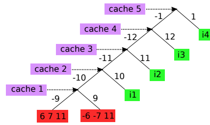
FIGURE 5 – Arbre de recherche pour marg2x2.cnf avec le cache.
