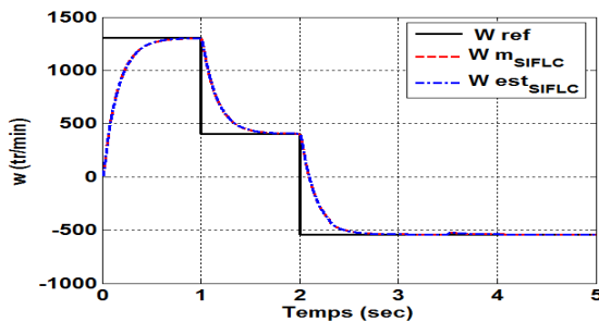
Figure. 21 : Allures des vitesses avec SIFLC, 2 e essai
