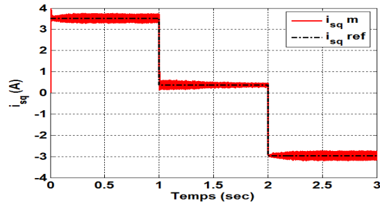
Figure. 11 : Courants statoriques quadratures (DRFOC-avec rotation de Park)
