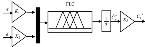
Figure.3 : le schéma bloc d'un contrôleur FLC standard
