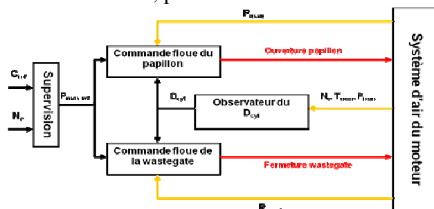
Figure 2 – Schéma général de contrôle du système d'air
