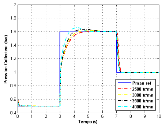
Figure 6 – Suivi de trajectoire de P_{man} en fonction de N_e
