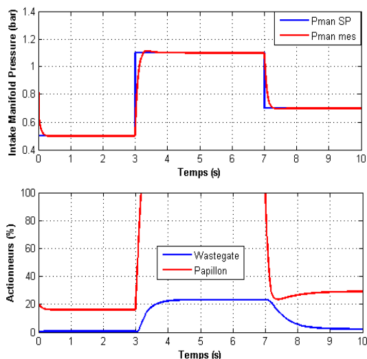
Figure 4 – Suivi de trajectoire P_{man} et commandes associées.
