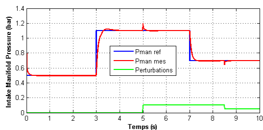
Figure 5 – Rejet de perturbations statiques
