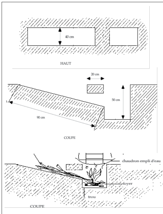
Fig. 74. Installation du kukuh nasi' , appareil à cuire le riz blanc en grandes quantité (croquis Pierre Le Roux, 1991, Pattani, Thaïlande du Sud).
