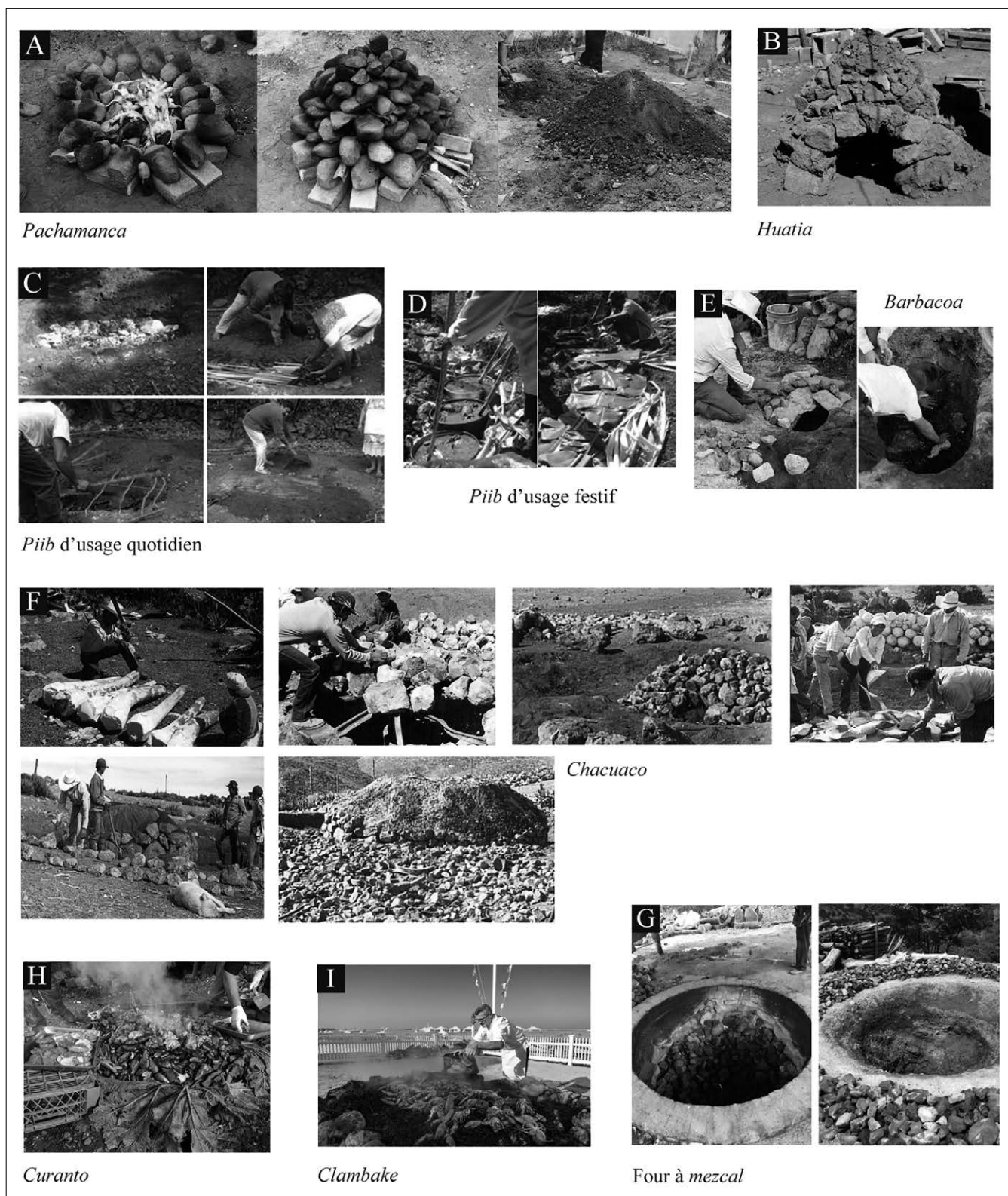
Fig. 11. Photographies de différents fours de terre mexicains et sud-américains contemporains (sources : A – photo Xauxa 2004 pour Wikicommons, CC-BY-SA ; B – Coraza Morveli, 2018, photo Arnold Fernandez Coraza) ; C – et D – Salazar et al. , 2012 ; fig. 3 et 4 ; E – Stark, 2002, fig. 8.1 et 8.35 ; F – Stark, 2002, fig. 4.5 à 4.11 ; G – Elixir of the Gods , 2018 ; H – Edible Adventure Travel, 2018, photo J. Mullin ; I – Chatham Bars Inn, 2021)
