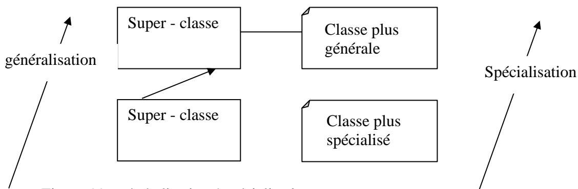
Figure 11 : généralisation / spécialisation
