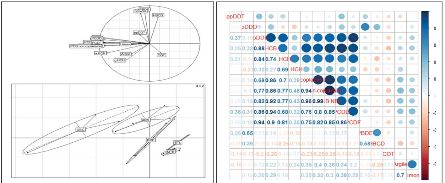
Figure 1 : Analyse en composante principale : synthèse des corrélations entre polluants organiques et ellipses de distributions à l'échelle du Rhône.
