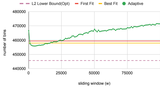
(d) Randomly_Generated benchmark from BPPLIB.
