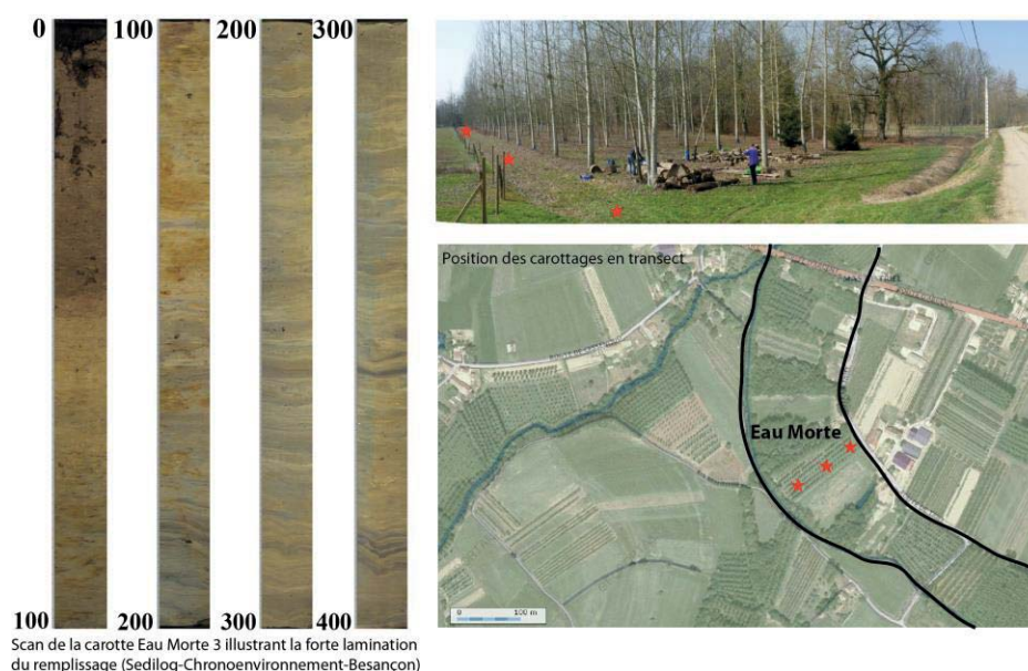
Fig. 1. Positionnement des carottages effectués dans le bras-mort de l'Eau Morte (Basses Terres Dauphinoises) et photos du remplissage micro-laminé.
