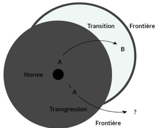
Figure 1 : Schéma de spatialisation des processus de transition et de transgression
