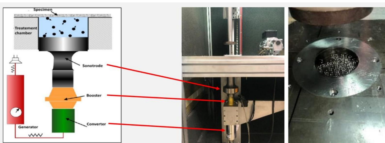
Figures 1,2,3 : Schéma du mécanisme SMAT [Ben Afia, 2016] (à gauche), photo de la machine SMAT du LASMIS (milieu), et photo de la chambre de traitement remplie de billes (droite) [Daban, 2022]
