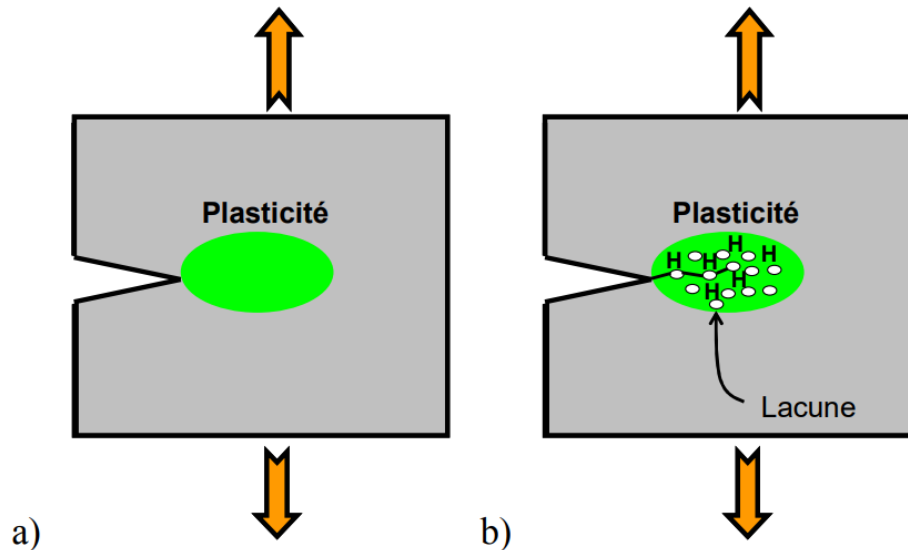
Figure 16 : Schématisation du mécanisme HESIVE, rupture sans hydrogène (a) et avec hydrogène (b), [Moro, 2009].
