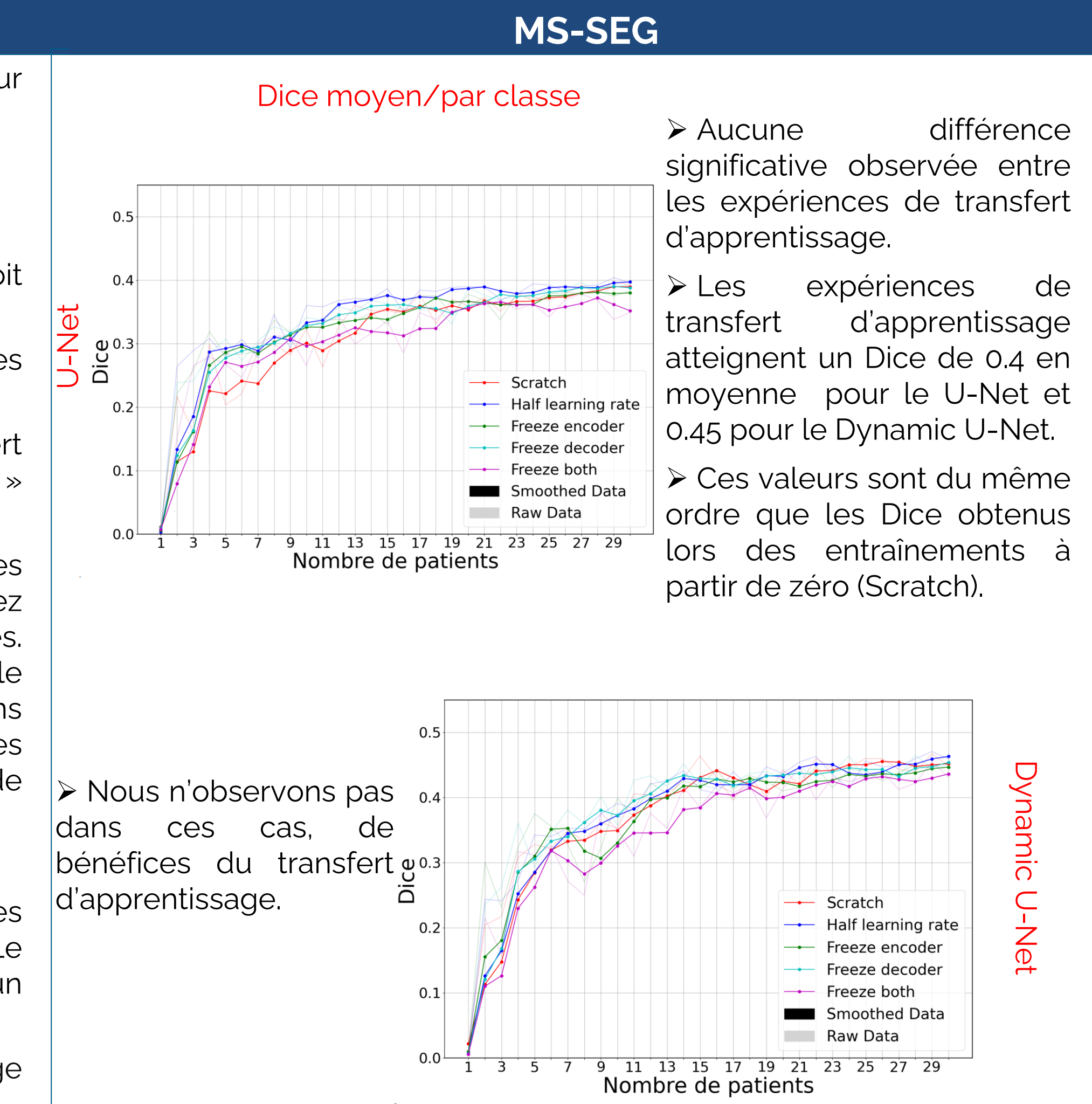
Figure 10: Dice obtenus avec les modèles U-Net et Dynamic U-Net sur la base de données MS-SEG.
