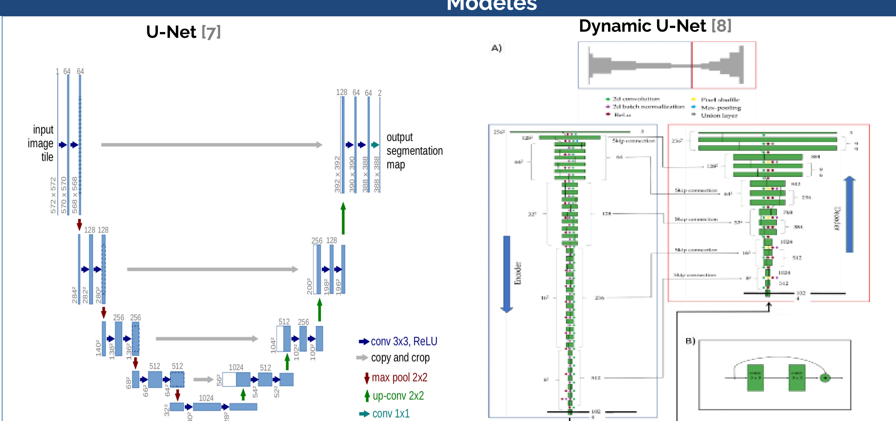
Figure 5: Architecture du réseau de neurones U-Net. Figure 6: Architecture du réseau de neurones Dynamic U-Net.
