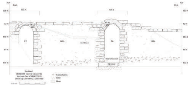
Figure 3: Elevation of wall 4. © S. Dhennin, J. Le Bomin
