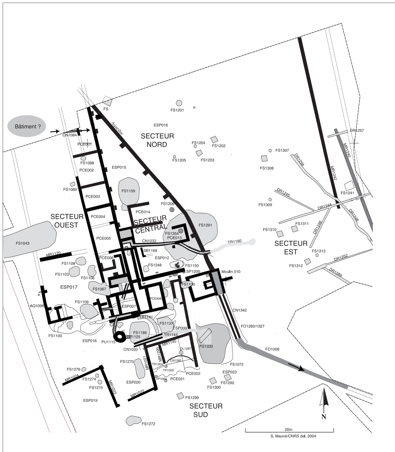
Fig. 2. Plan général des vestiges et constructions mis au jour lors de la fouille de L'Auribelle-Basse (2001-2004). Relevé G. Marchand, S. Mauné, J.-P. Martinez. DAO S. Mauné. Éch. 1/500°
