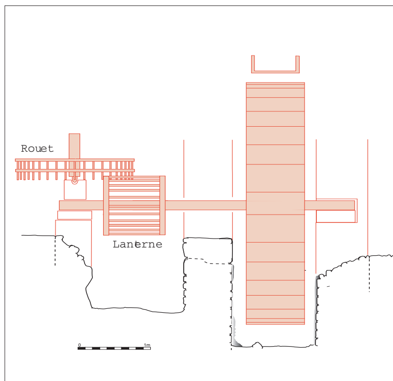
Fig. 22. Proposition de restitution en coupe du mécanisme de l'état 1 du moulin hydraulique de L'Auribelle-Basse (Pézenas, Hérault). Dessin J.-L. Paillet, DAO R. Bourgaud et S. Mauné Éch. 1/50°
