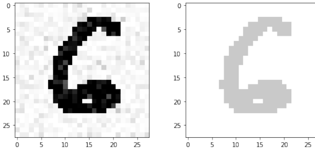
FIGURE 2.5 – Comme la condition d'irreprésentabilité n'est pas satisfaite pour la matrice particulière X et le schéma \beta , l'estimateur SLOPE \hat{\beta}_{\gamma_{\text{surre}}} est peu susceptible de récupérer le schéma \beta . En effet, le graphique de gauche montre que \hat{\beta}_{\gamma_{\text{surre}}} , redimensionné comme une image de taille 28 \times 28 , ne récupère pas le schéma \beta . En revanche, la condition d'accessibilité est satisfaite et donc l'estimateur SLOPE seuillé peut révéler le schéma \beta . En effet, le graphique de droite illustre que \text{prox}_{\tau\lambda}(\hat{\beta}_{\gamma_{\text{surre}}}) , redimensionné comme une image de taille 28 \times 28 , récupère le schéma \beta (ici, \tau > 0 est le plus petit nombre réel pour lequel \text{prox}_{\tau\lambda}(\hat{\beta}_{\gamma_{\text{surre}}}) a un unique groupe d'appariement non-nul).
