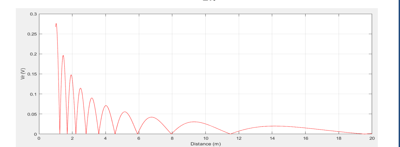
Tension reçue au niveau du récepteur (configuration 1LOS+1NLOS)
