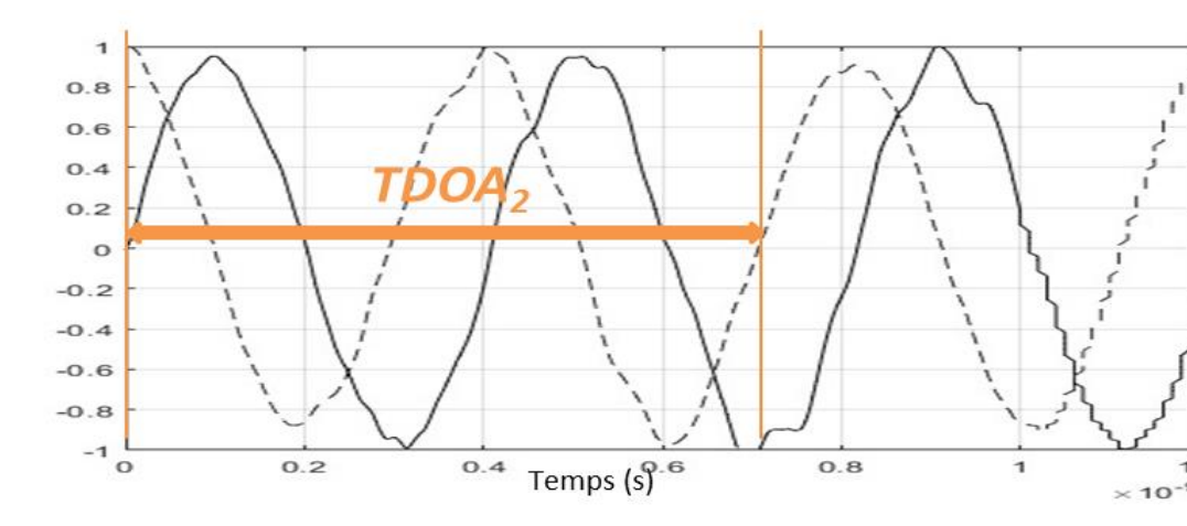
TDOA 2 entre les récepteurs A 1 et A 3
