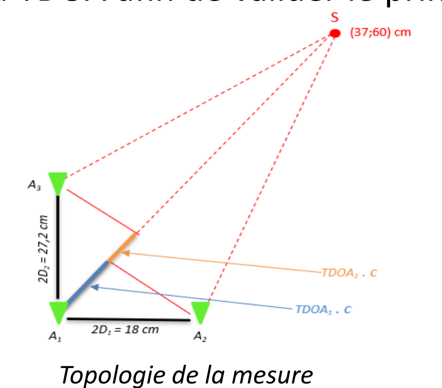
Topologie de la mesure
