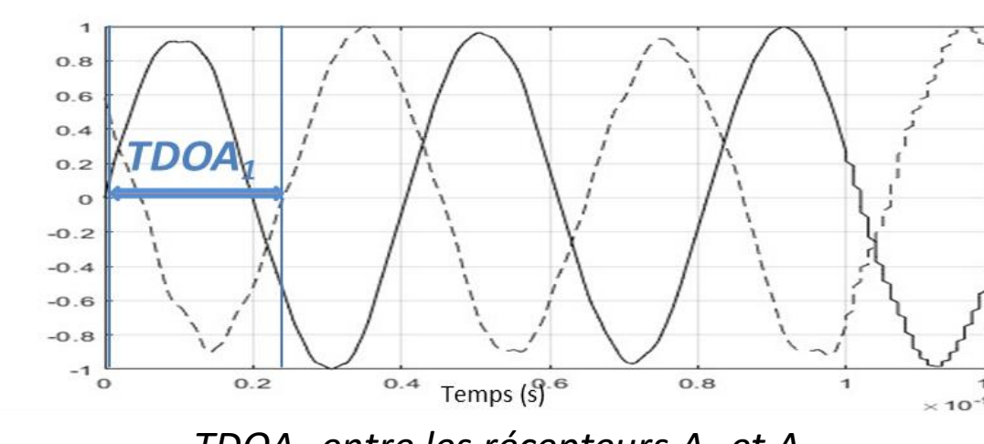
TDOA 1 entre les récepteurs A 1 et A 2
