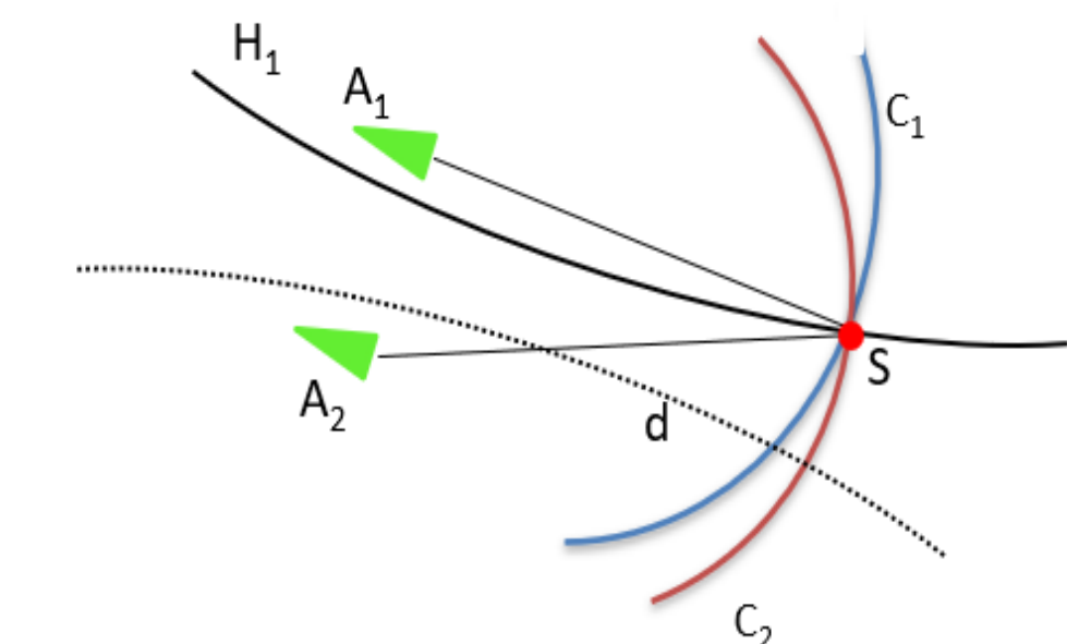
Schéma de la localisation par fusion TDOA/RSS
