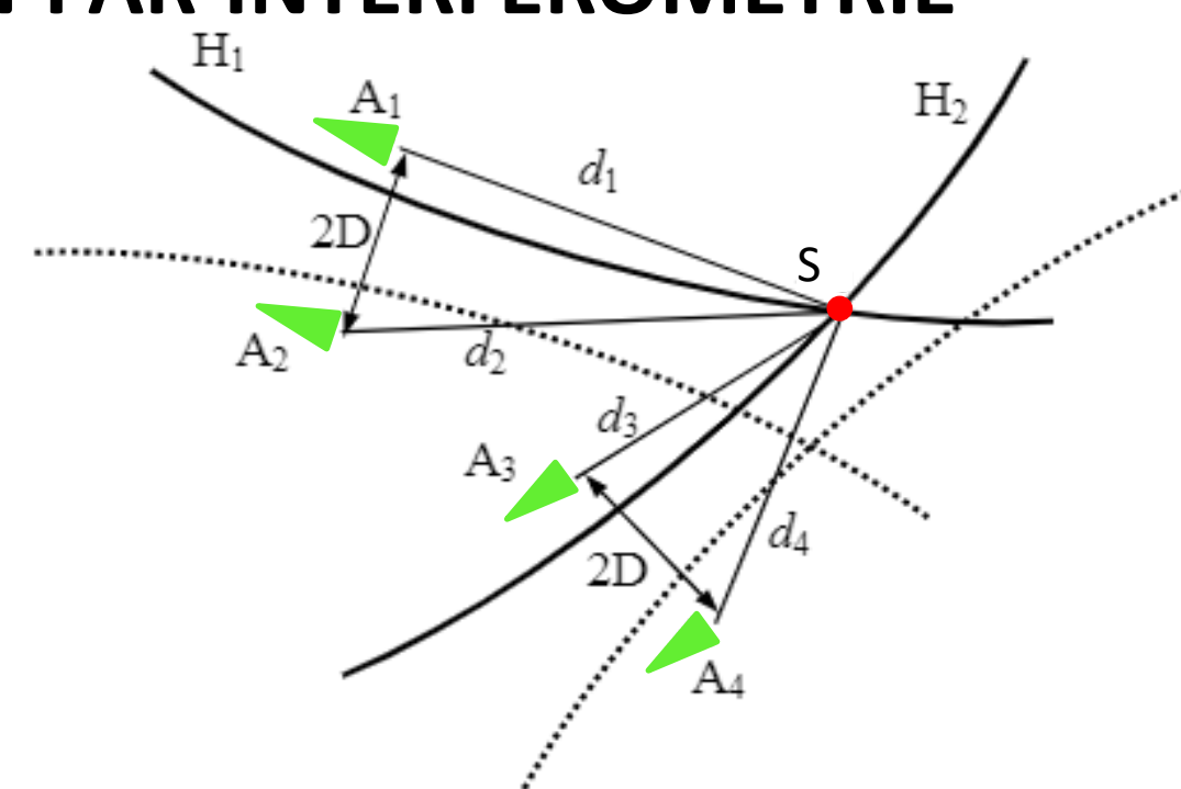
Schéma de la localisation interférométrique
