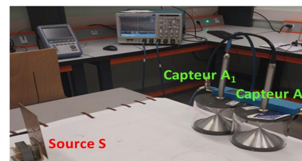
Source: antenne patch à 2,45GHz Capteurs: antennes Biconiques (400MHz - 8GHz)
