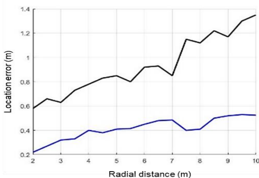
Figure 7. Erreur de localisation Vs distance radiale (courbe noire : D = 10cm ; courbe bleue : D = 50 cm)
