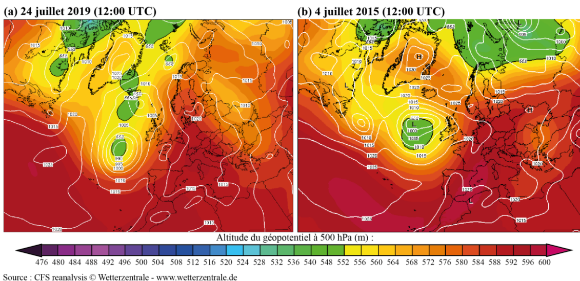
Figure 3. Cartes du champ de pression de surface (contours blancs ; hPa) et de l'altitude du géopotential à 500 hPa (plage de couleurs ; m) sur le secteur Atlantique Nord – Europe à 12:00 UTC (a) le 24 juillet 2019 et (b) le 4 juillet 2015. Source : Wetterzentrale ( www.wetterzentrale.de ), réanalyse CFS. Maps of surface pressure (white contours; hPa) and 500 hPa geopotential height (shadings; m) over the North Atlantic – Europe sector at 12:00 UTC in (a) July 24, 2019 and (b) July 4, 2015. Source: Wetterzentrale ( www.wetterzentrale.de ), CFS reanalysis.
