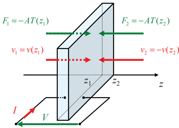
Figure 1: Modélisation de Mason d'une couche piézoélectrique.
