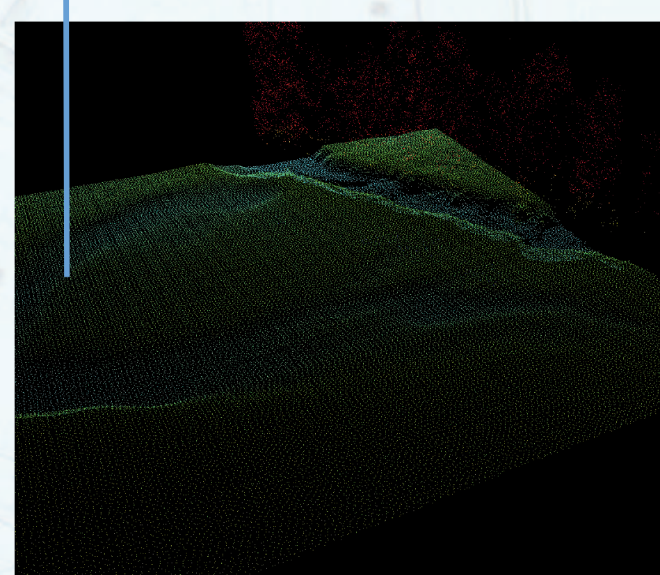
PCA
