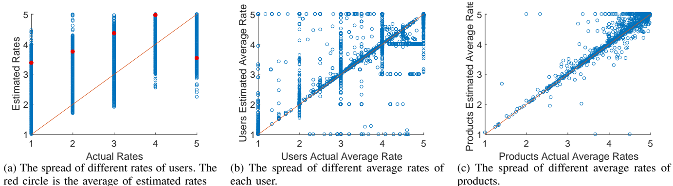
Fig. 4: Etsy dataset
