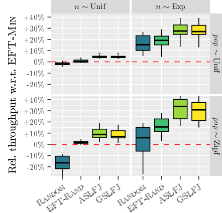
(b) Relative throughput w.r.t. EFT-MIN.
