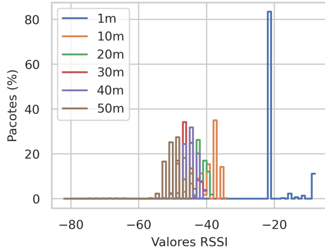
Figura 6. Distribuição de valores RSSI para diferentes distâncias.
