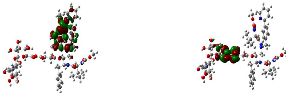
Figure 3 (c) HA-Atazanavir HOMO orbital (d) HA-Atazanavir LUMO orbital
