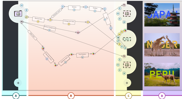
Fig. 2 – [  gauche] Interface du logiciel CAT pour la "Conception d'un template". De gauche   droite : (A) les ressources du template; (B) l'espace de composition des r gles du template; (C) les emplacements texte/image de la mise en page, (D) le rendu du template avec les 3 mises en pages g n r es en simultan es. [  droite] un exemple d'incrustation du texte dans l'image propos e par Mathilde
