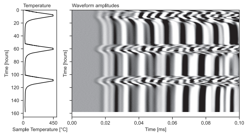
c) La Lumbre Basalt
