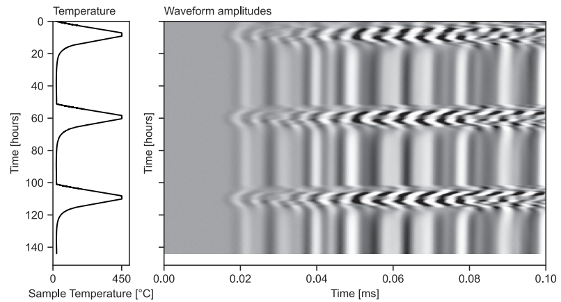
b) Rubble Creek Basalt
