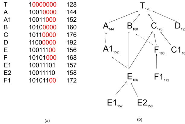
Fig. 1. LiteMat Encoding
