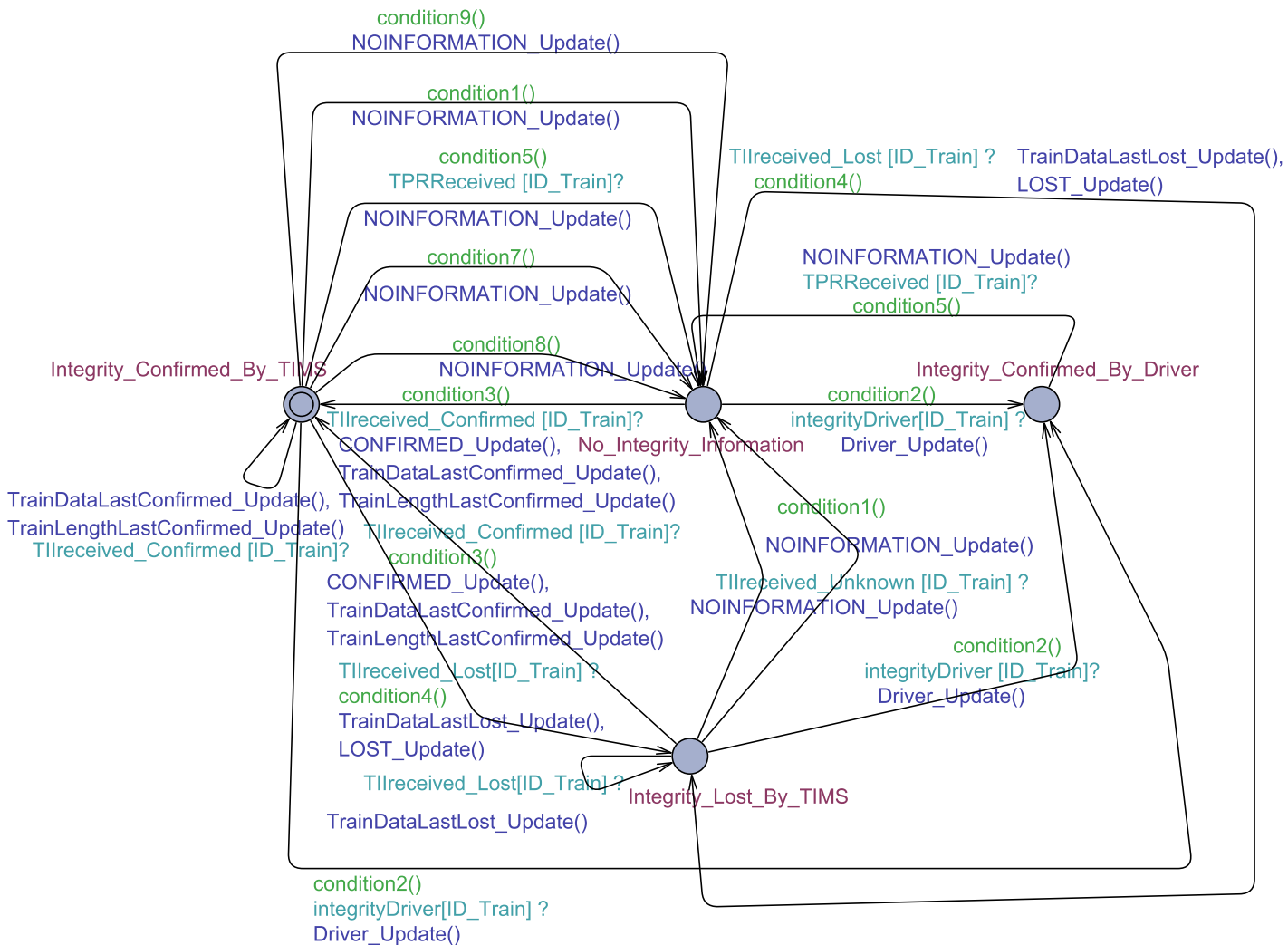
Fig. 4.8. IIM_StatusManagement automaton
