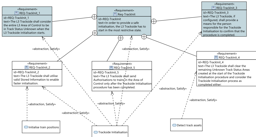
Fig. 6.12. The Trackside Initialization EUC RD
