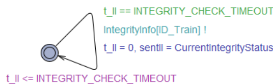
Fig. 8.9. IIM updating automaton
