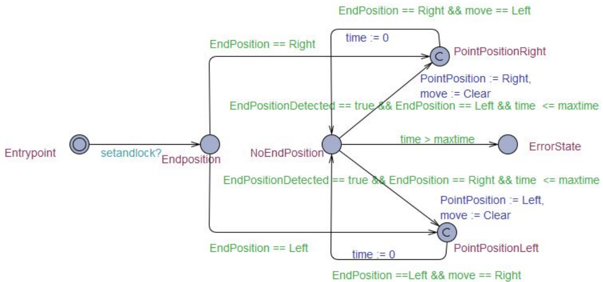
Fig. 8.15. SetandLock automaton
