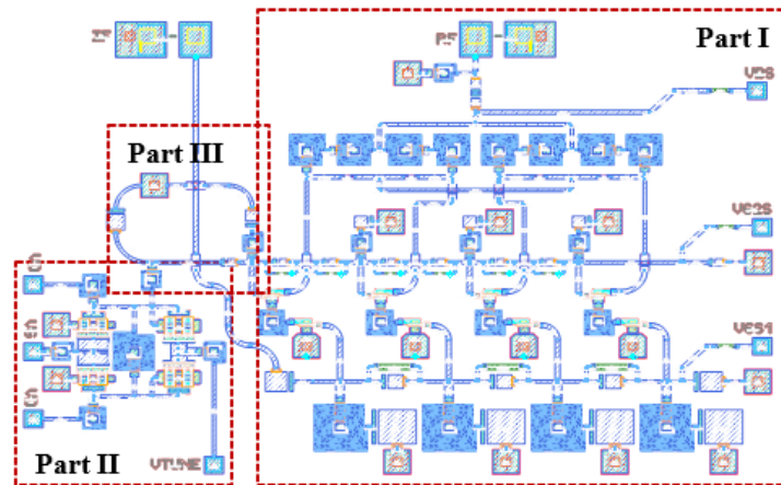
Figure 8. 5G mm-wave SOM layout
