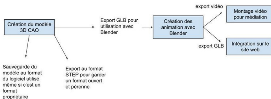
Figure 3: Processus de création 3D de CHRONOSPEDIA
