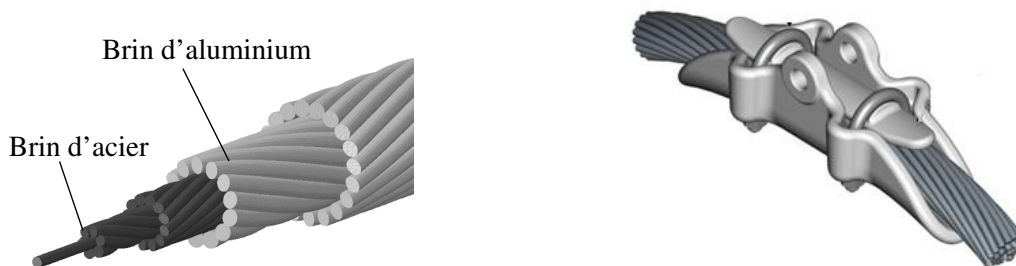
(a) Représentation schématique d'un conducteur ACSR
