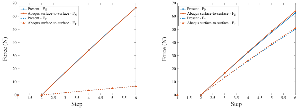
(a) Efforts de contact pour un coefficient de frottement de 0.1 (b) Efforts de contact pour un coefficient de frottement de 0.8
